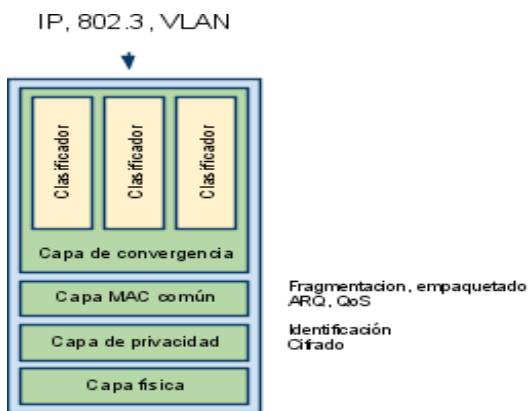
Figura 6 - Modelo de referencia en aerDOCSIS
