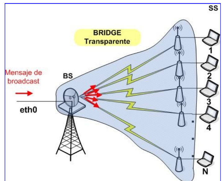
Figura 7 - Modo Bridging
