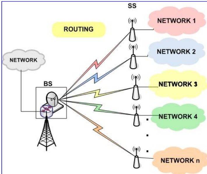
Figura 8 - Modo Routing
