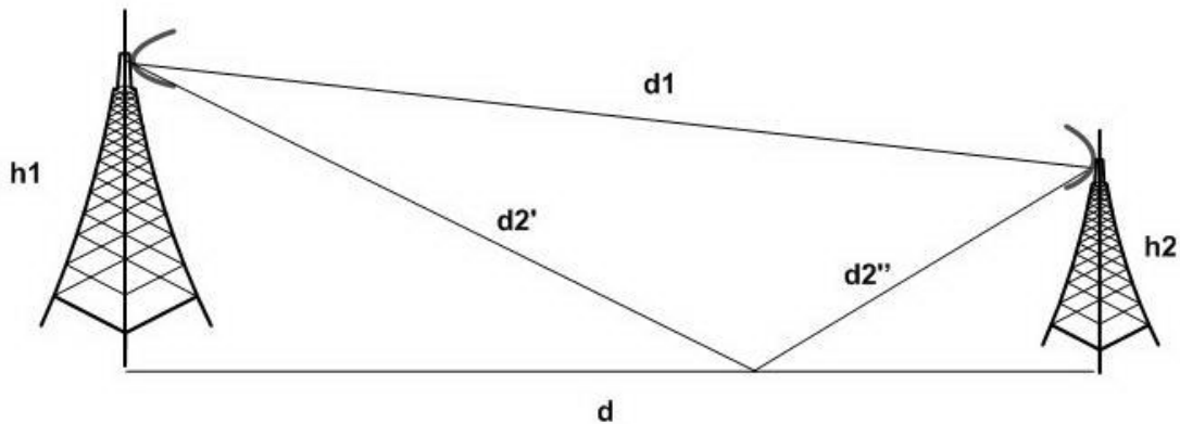
Figura 5 - Modelo simple de rayo reflejado
