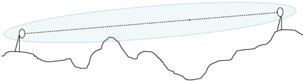
Figura 3 - Despejamiento parcial (> 60%) de la 1ª zona de Fresnel
