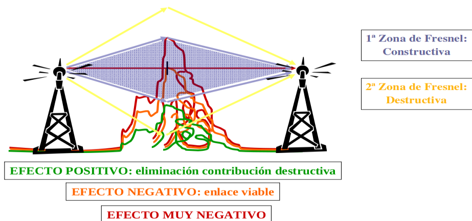
Figura 1 - Efecto de los obstáculos sobre las zonas de Fresnel
