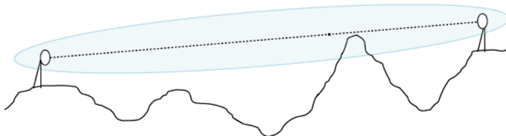
Figura 4 - Obstrucción de la 1ª zona de Fresnel
